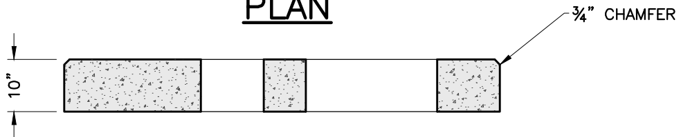
SECTION A-A
